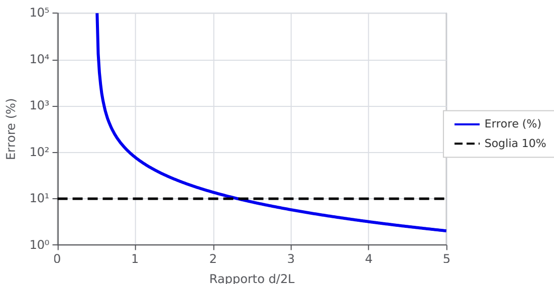
Figura 2. Errore relativo di misura nel caso 3 (attenuazione 1/r^3 ), in funzione della distanza d del centro del sensore dal conduttore sorgente, normalizzata al lato 2L del sensore stesso.
