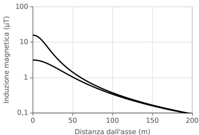
Figura 6. Profilo laterale dell'induzione magnetica ad 1 metro dal suolo, generata da un elettrodotto semplice terna 380 kV/1500 A con sostegni standard a traliccio; curva superiore: conduttore più basso a 15 metri dal suolo; curva inferiore: conduttore più basso a 35 metri dal suolo
