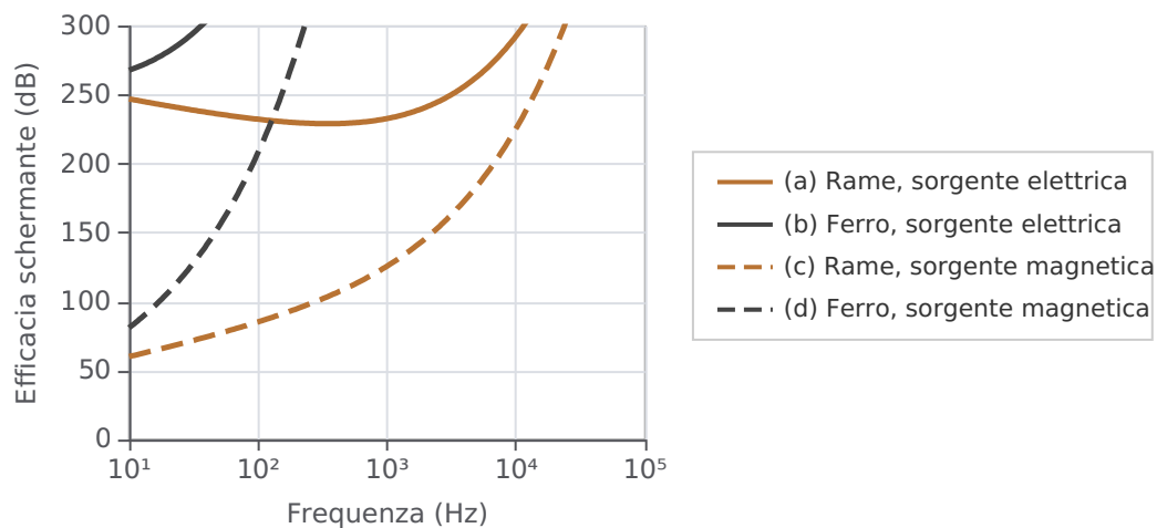
Figura 2. Efficacia schermante di una lastra di rame (linee (a) e (c)) e di ferro (linee (b) e (d)) in funzione della frequenza da 10 Hz a 100 kHz. La lastra ha uno spessore di 1 cm e si trova a 100 m da una sorgente di campo elettrico (linee (a) e (b)) o di campo magnetico (linee (c) e (d))
