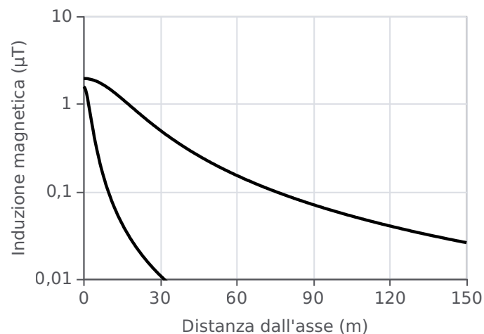
Figura 4. Profilo laterale dell'induzione magnetica ad 1 metro dal suolo, generata da un elettrodotto semplice terna 132 kV/450 A; curva superiore: linea aerea con sostegni standard a traliccio e conduttore più basso posto a 18 metri dal suolo; curva inferiore: linea interrata a trifoglio con il centro del trifoglio posto ad una profondità di circa 1.5 metri
