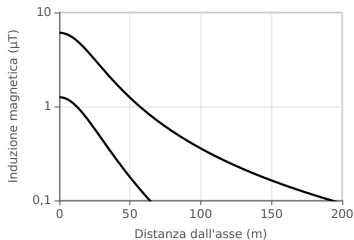
Figura 5. Profilo laterale dell'induzione magnetica ad 1 metro dal suolo, generata da linee a 380 kV/1 MW con sostegni standard a traliccio e conduttore più basso posto a 25 metri dal suolo; curva superiore: linea a semplice terna (corrente 1500 A); curva inferiore: linea a doppia terna ottimizzata (corrente 750 A)
