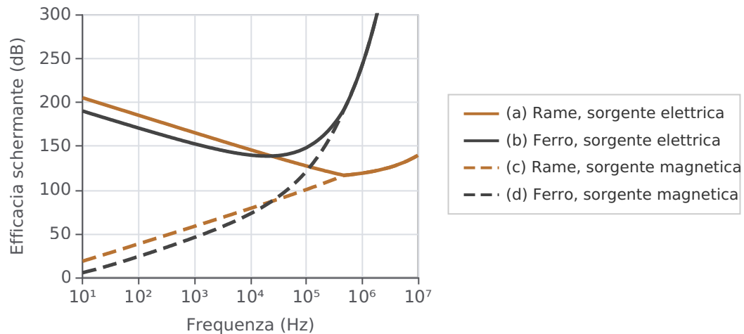
Figura 1. Efficacia schermante di una lastra di rame (linee (a) e (c)) o di ferro (linee (b) e (d)) in funzione della frequenza da 10 Hz a 10 MHz. La lastra ha uno spessore di 0.1 mm e si trova a 100 m da una sorgente di campo elettrico (linee (a) e (b)) o di campo magnetico (linee (c) e (d))
